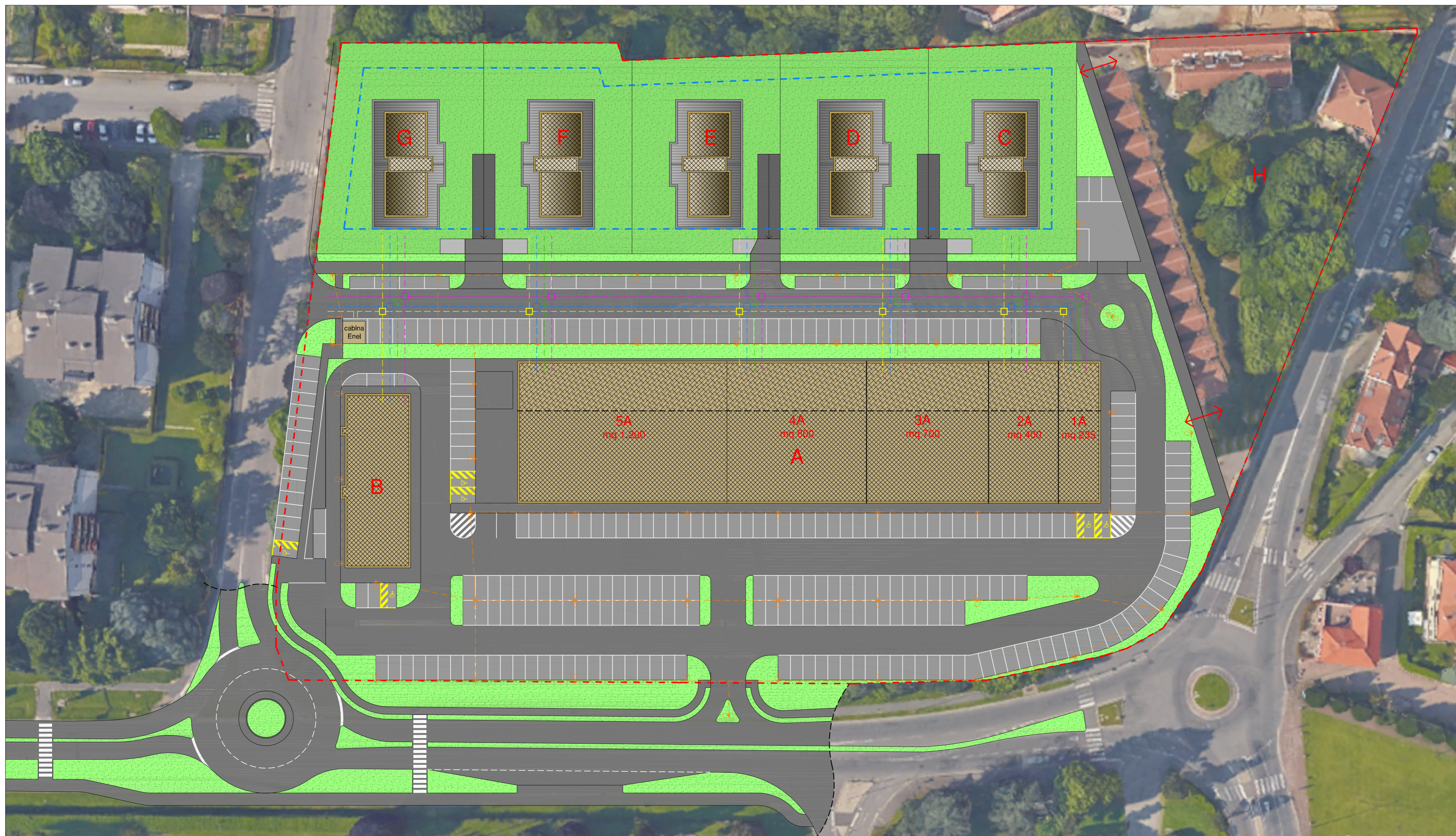
PLANIMETRIA (Reti Tecnologiche) - scala 1:500
