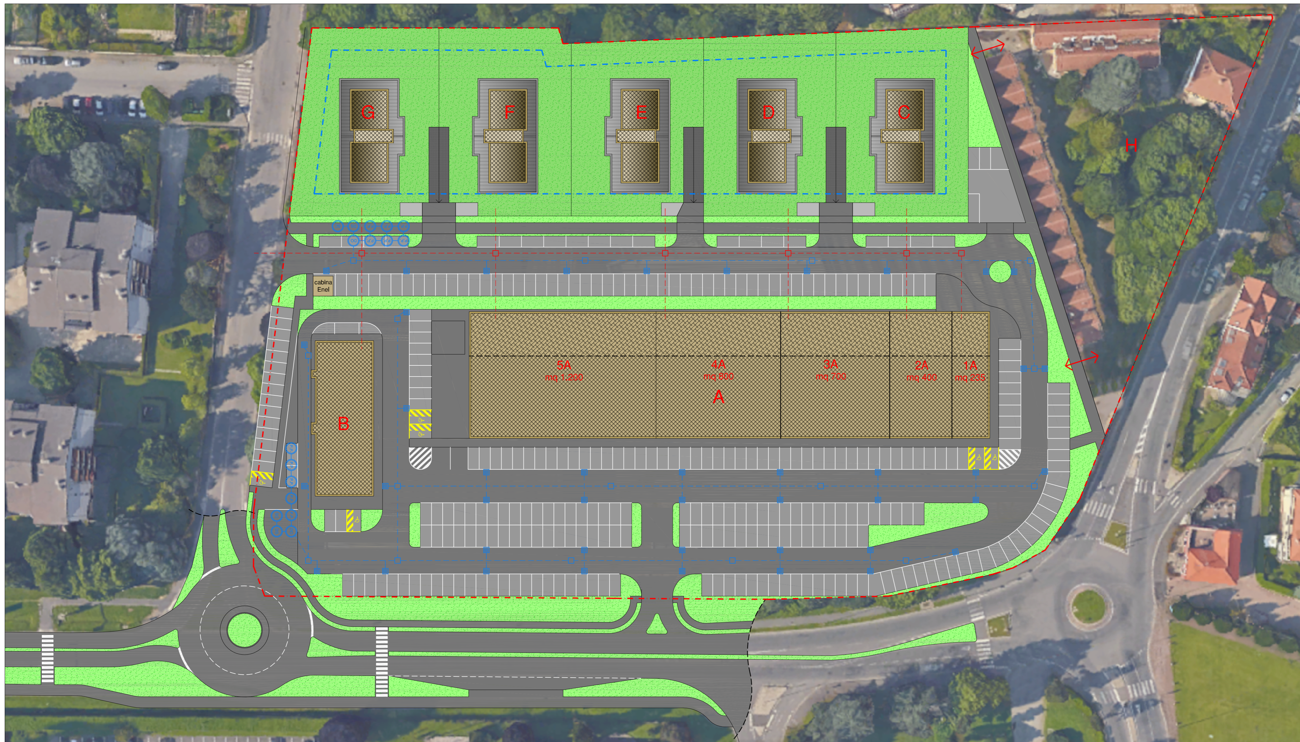
PLANIMETRIA (Schema di fognatura) - scala 1:500
